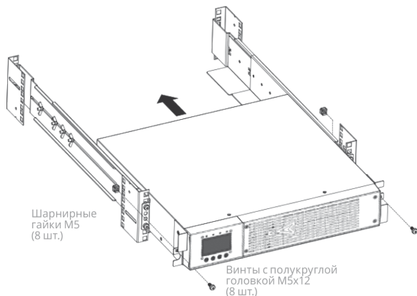
Рисунок 3.2. Крепление ИБП в стойке
